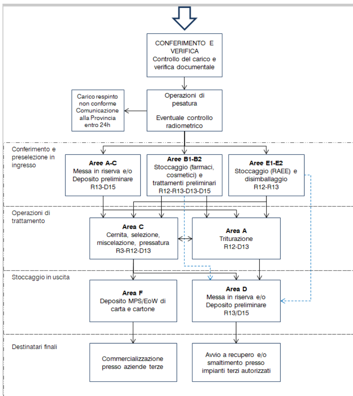
Figura B8 – Schema del processo produttivo
